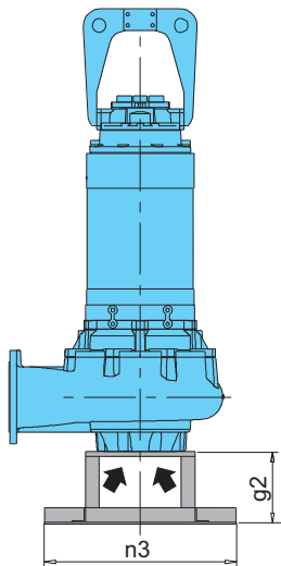
Модификация со стойкой и коленом 90°
